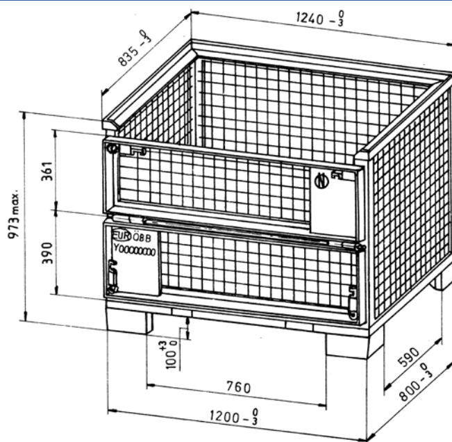
Gitterboxpalette UIC Norm 435/3
